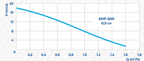
CURVA CARACTERÍSTICA
