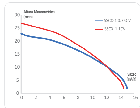
Comparativo curvas HxQ
